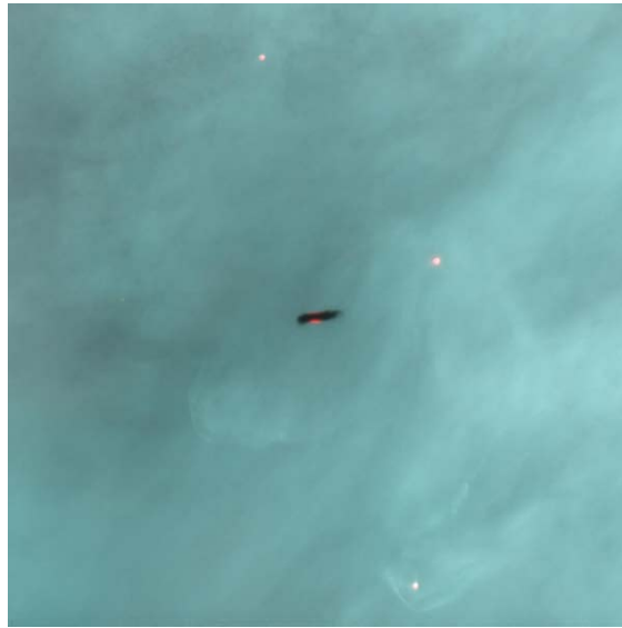
Figuur S.2 — Een afbeelding in het visuele bereik van de zijkant van een protoplanetaire schijf, genomen met Hubble. Het stof in de schijf blokkeert de straling van het gas en stof in de achtergrond. Dit is een vergelijkbare afbeelding zoals genomen in 1993 door O'Dell, die het cruciale bewijs vormde voor accretieschijven rond jonge sterren. Credits: J. Bally (Universiteit van Colorado) en H. Throop (SWRI).
